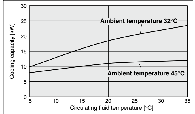
HRL□-A/W□-40-T2 (CH2)*2
