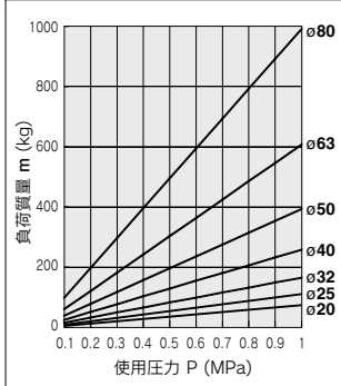
グラフ 5 ~500mm/s
