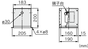
仕様表
