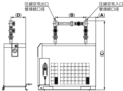
寸法表 (mm)
