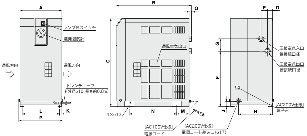
寸法表
