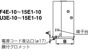
寸法表 (mm)
