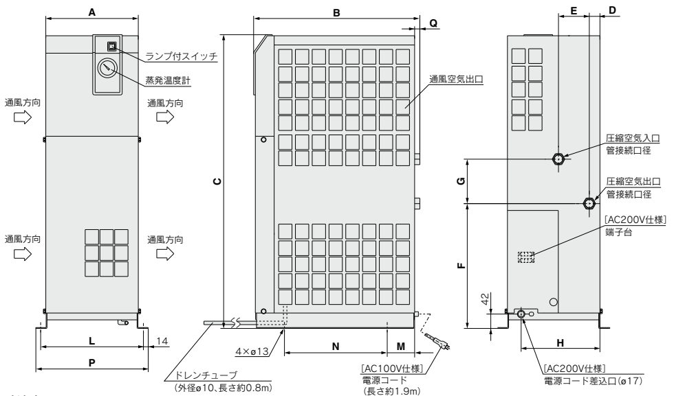
寸法表
