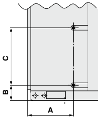
寸法表 (mm)
