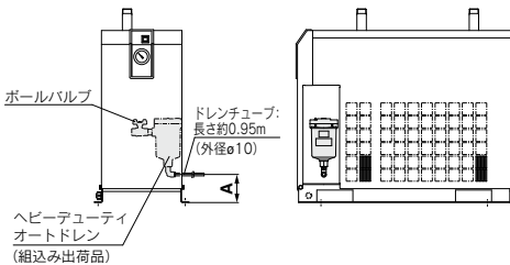
寸法表 (mm)
