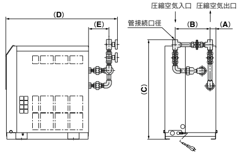
寸法表 (mm)
