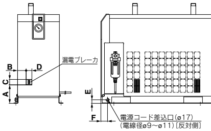
寸法表
