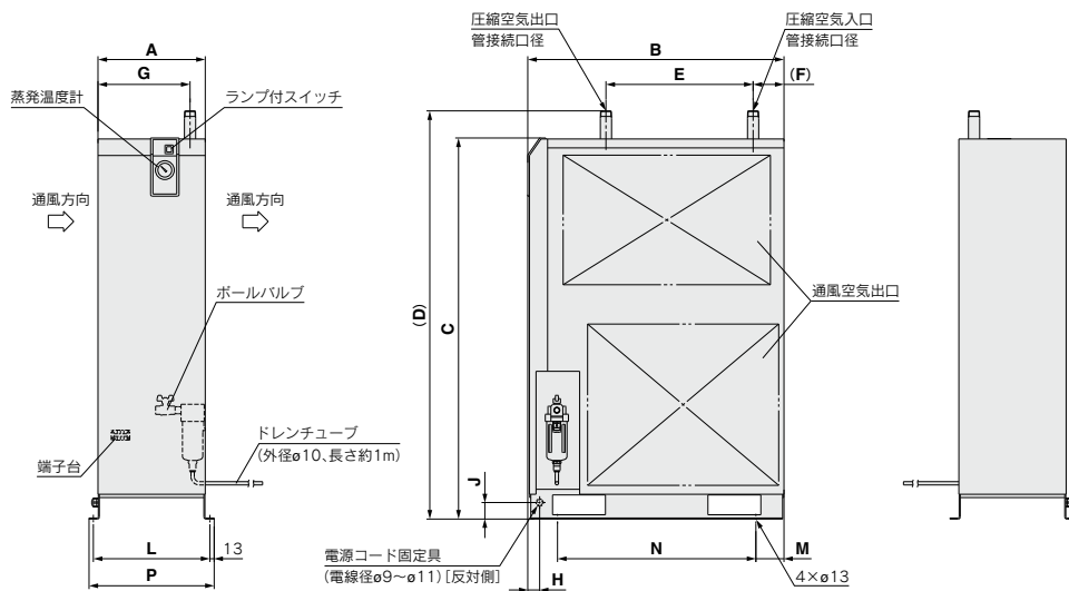
寸法表
