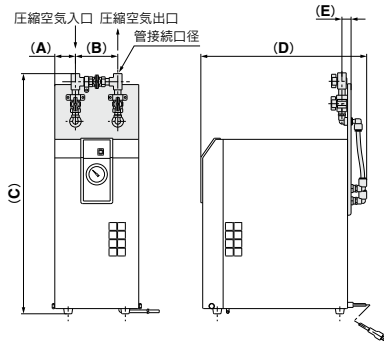
寸法表 (mm)
