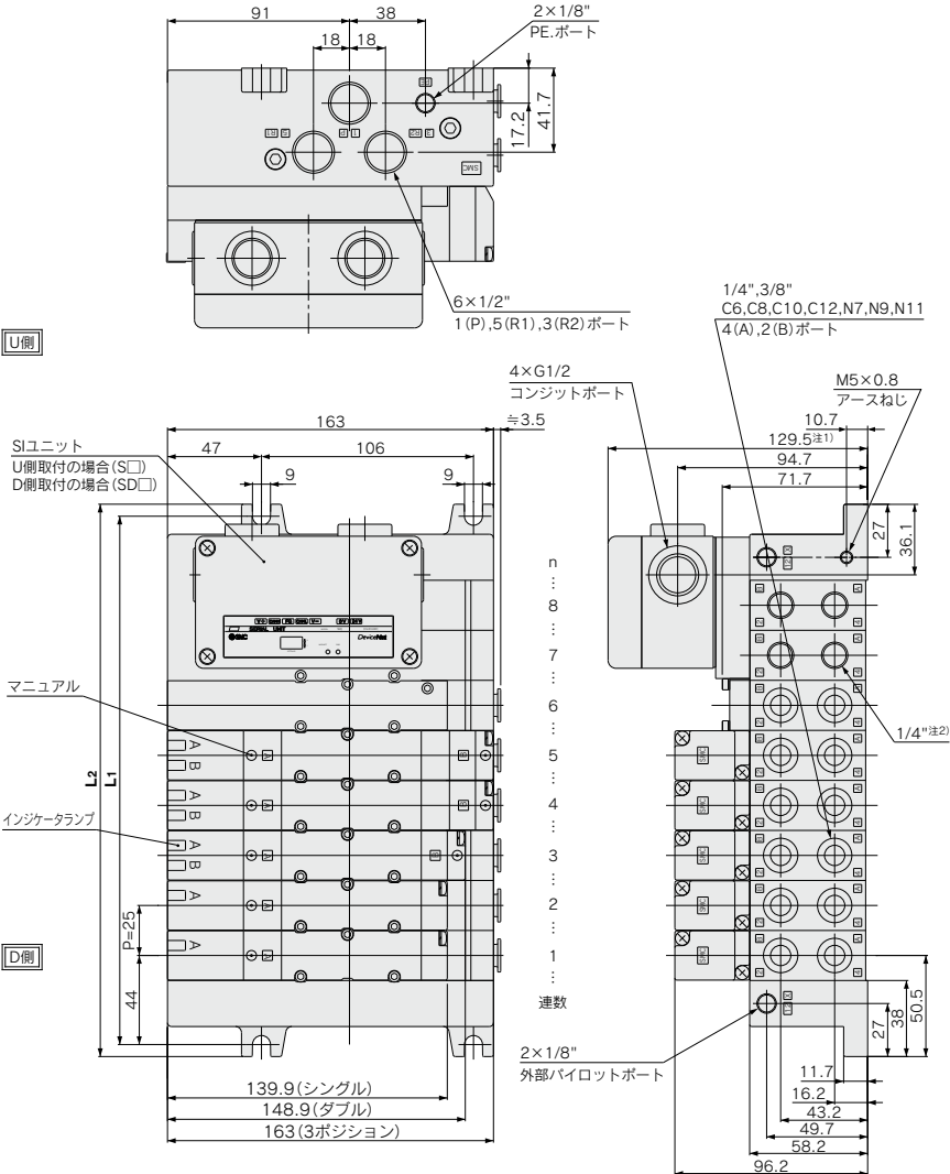
図はVV5Q41-08C12SQ-Wを示す。
