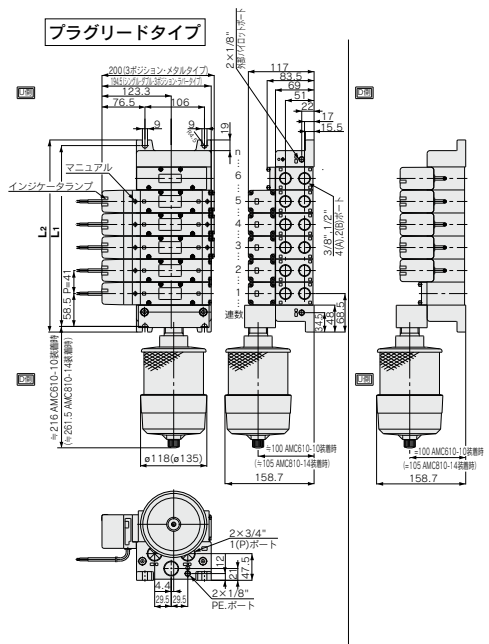
寸法表 計算式 L_1=41n+76 L_2=41n+96 n: 連数(最大12連)
