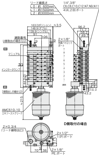
寸法表 計算式 L1=25n+63 L2=25n+76 n: 連数(最大16連)
