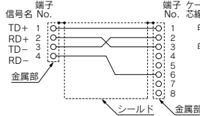
結線図(ストレートケーブル)
